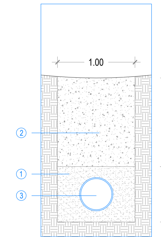
SEZIONE TIPO scala 1:20
